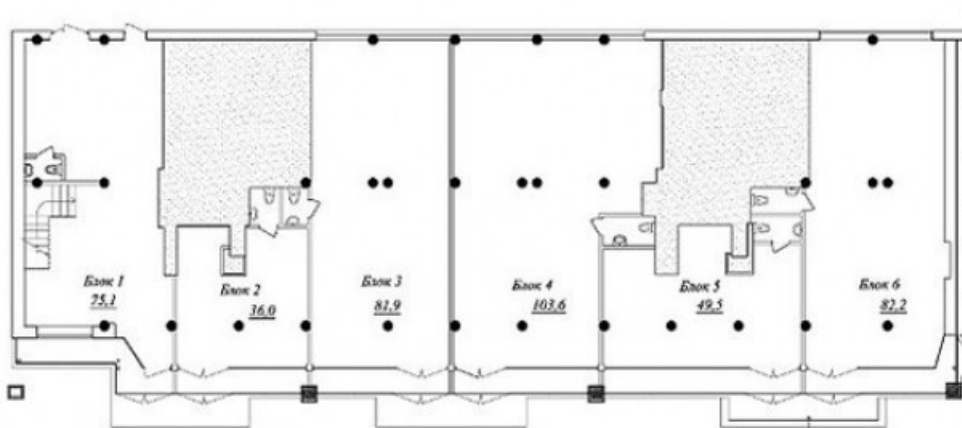
План подвала
