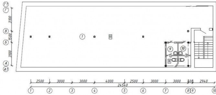
План эксплуатируемого чердака
