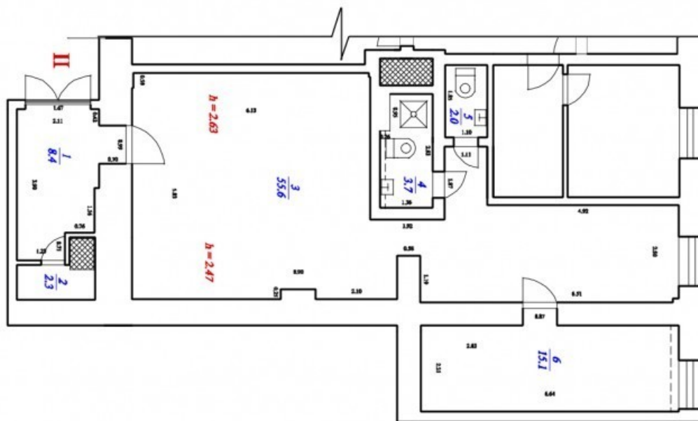
План 1 этажа
