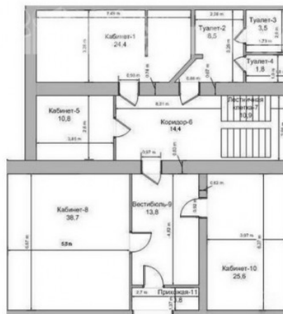
1Й ЭТАЖ
