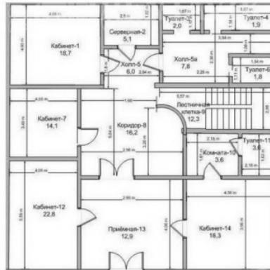
3Й ЭТАЖ
