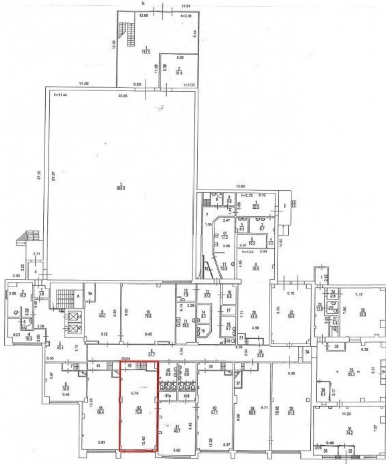
1-й этаж
