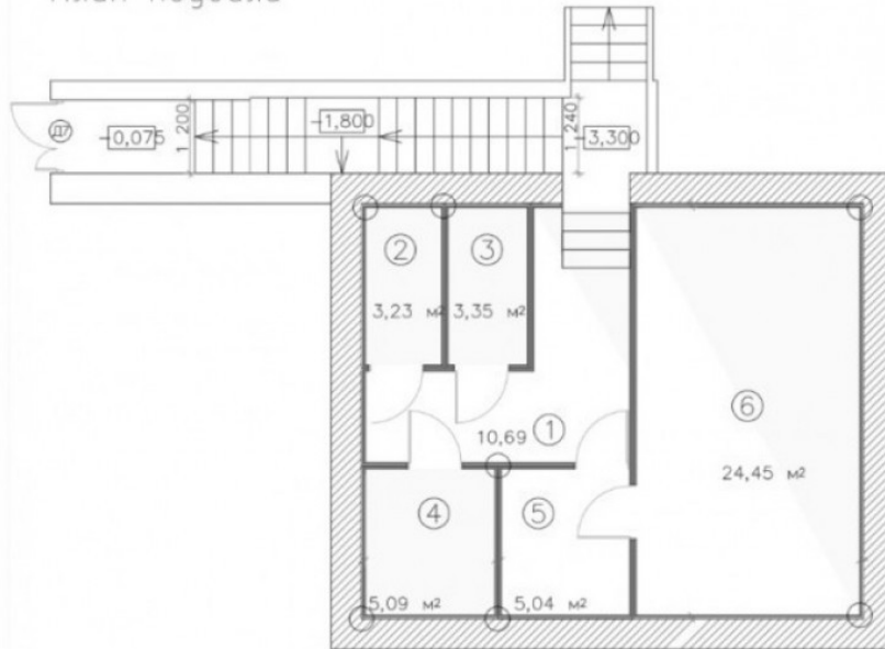
План подвала
