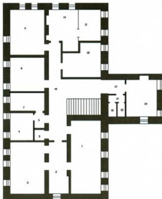
План 2-го этажа Общая площадь 306,4 кв. м.
