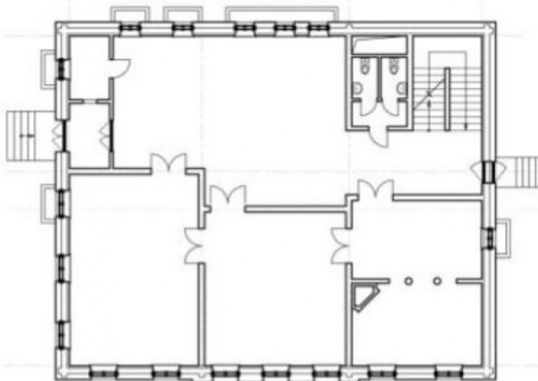
План 1-ого этажа.
