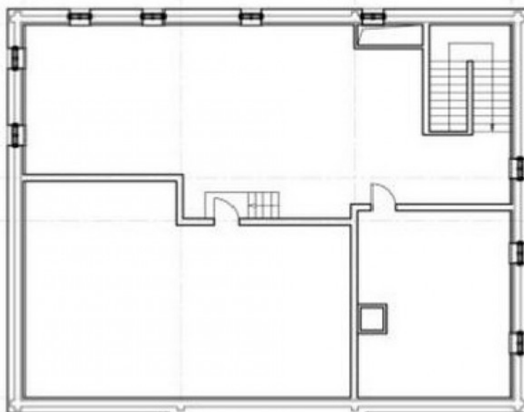
План подвала.
