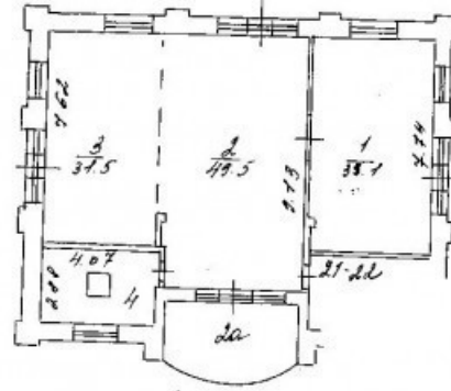
2 й ЭТАЖ
