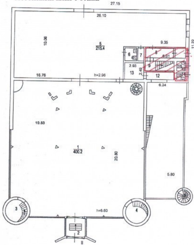
Поэтажный план 1 этажа
