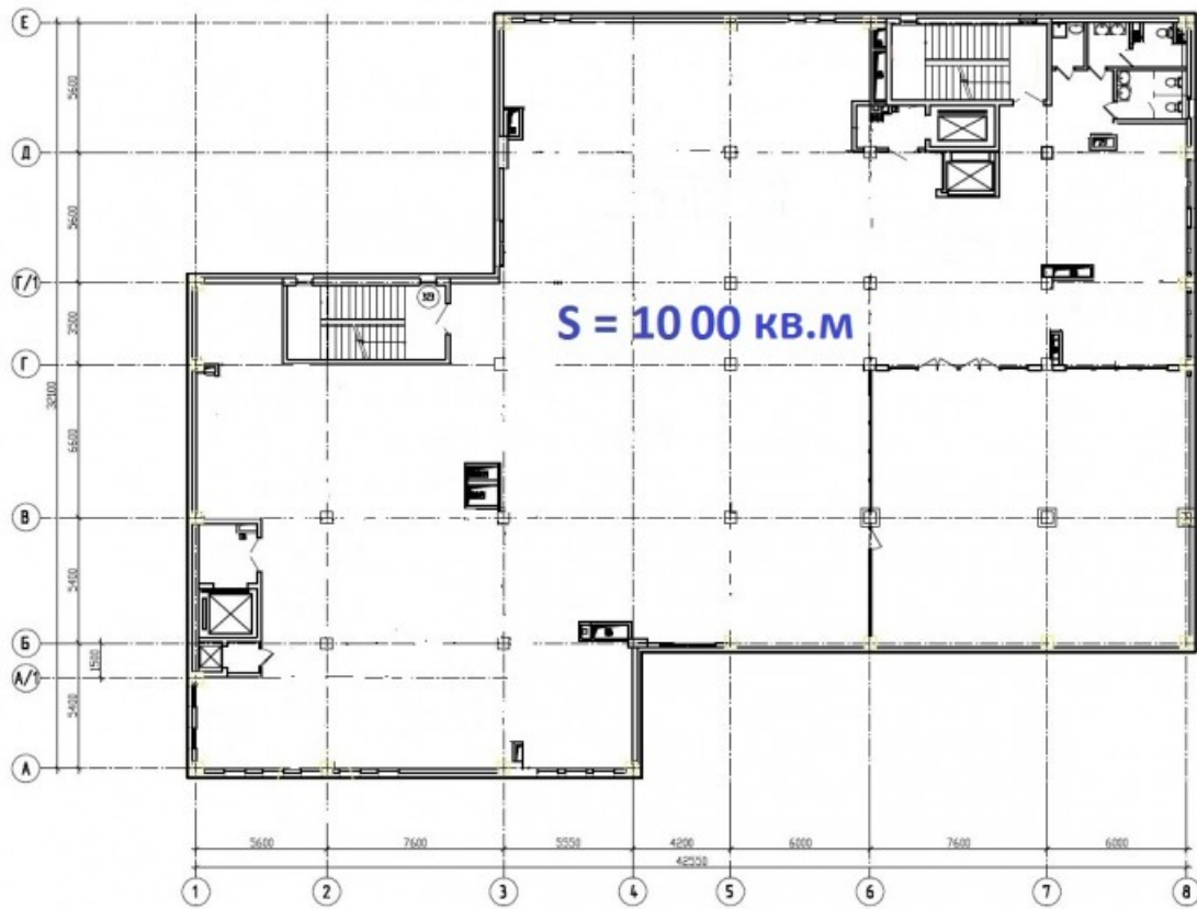
План 3 этажа
